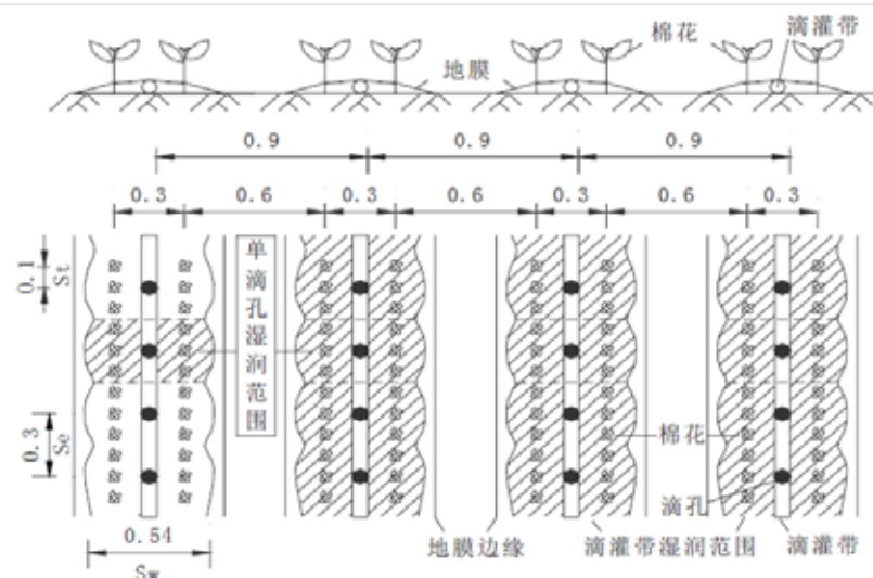
图2.2 滴灌带与作物布置简图
