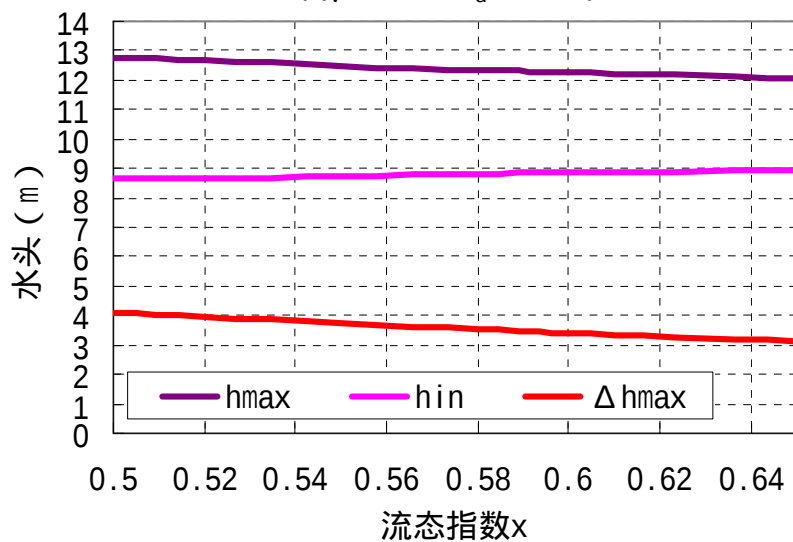
不同流态指数 x 对灌水小区最大水头偏差的影响 ( q_v=0.2 h_d=10\text{m} )
