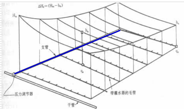
图 4-28 灌水小区的压力水头分布图
