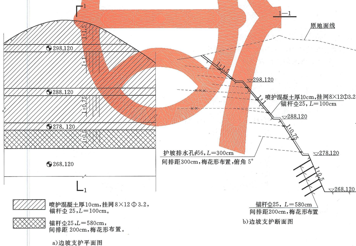
图 4.2.10-2 边坡支护图
