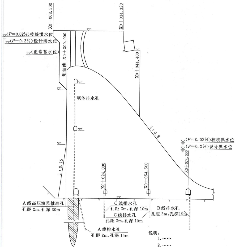
图 4.2.11-2 帷幕灌浆图
