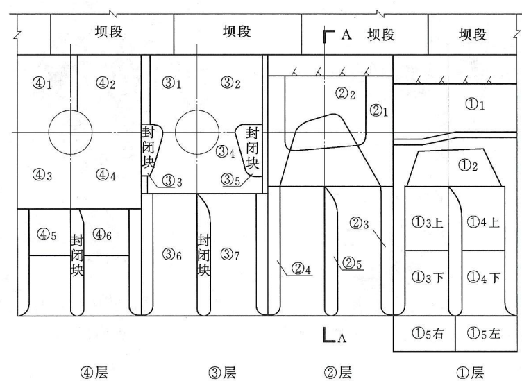
a) 厂房机组段分层分块平面图
