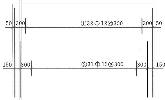
图 4.3.11 相间排列钢筋的简化画法
