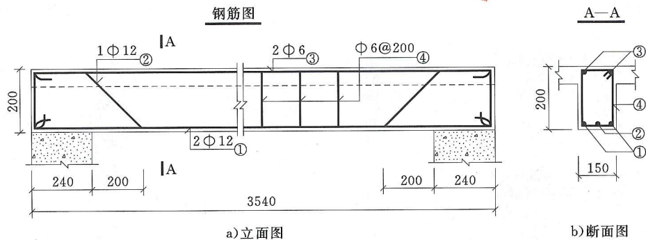
图 4.3.1 钢筋图
