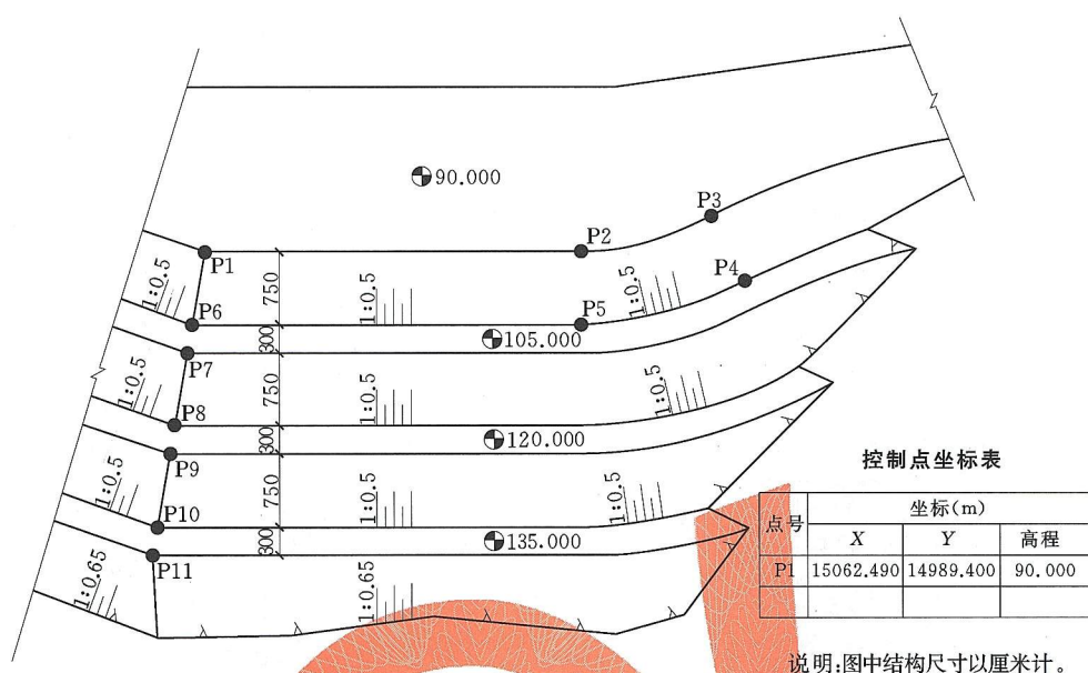
图 4.2.10-1 开挖平面图
