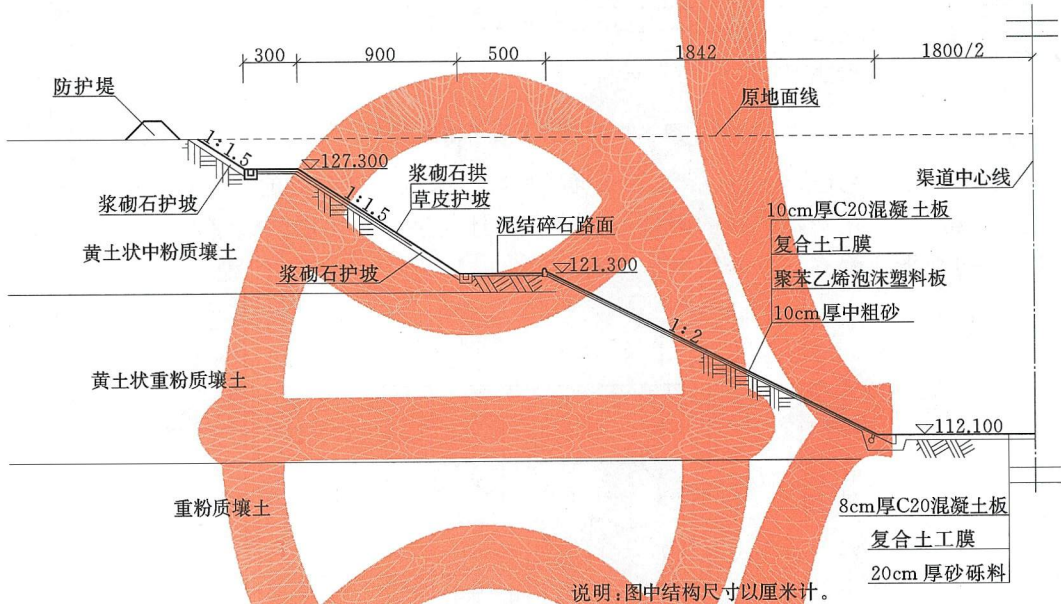
图 4.2.9-4 渠道断面图
