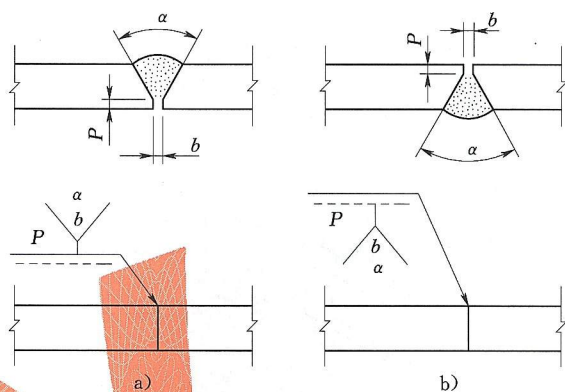
图 5.4.2 单面焊缝的标注
