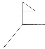
图 5.4.9 现场焊缝标注
