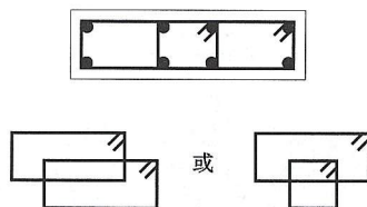
图 4.3.5-4 箍筋详图
