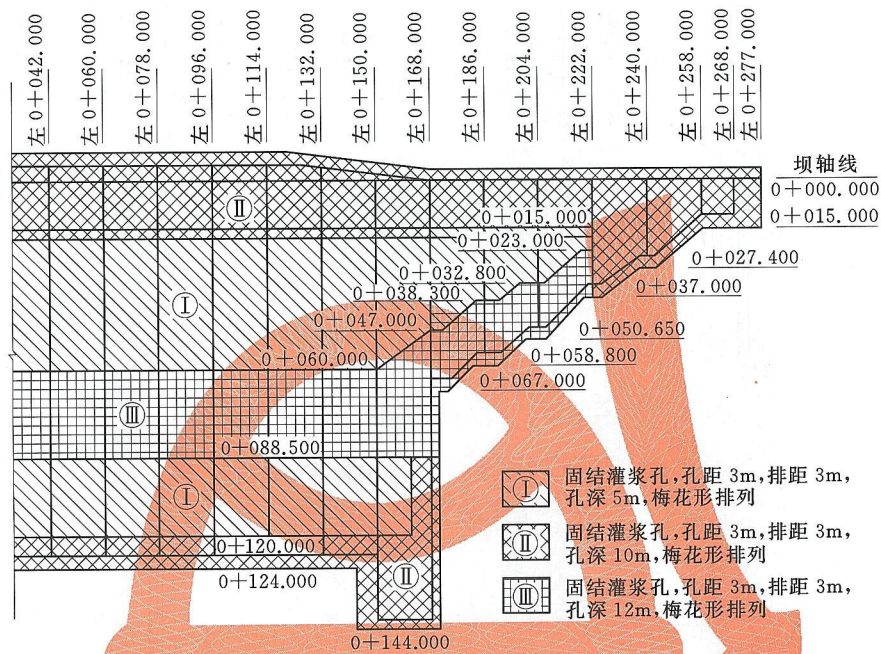
图 4.2.11-3 固结灌浆图
