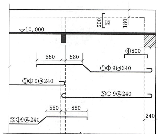
图 4.3.6 板类构件平面图中的钢筋表示法
