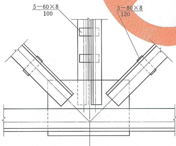
图 5.3.2 节点图
