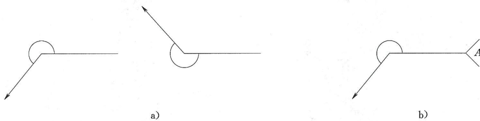
图 5.4.10 相同焊缝标注
