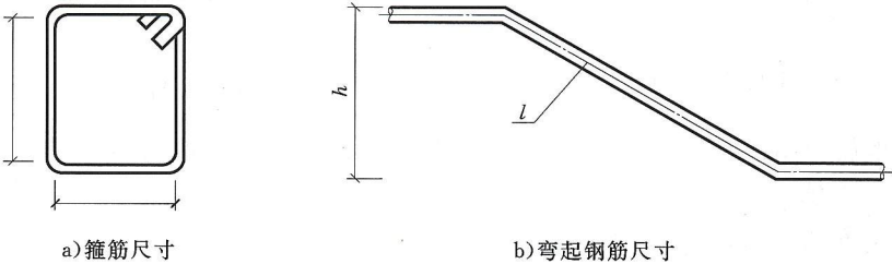
图 4.3.3-2 箍筋和弯起钢筋尺寸
