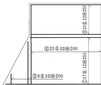
图 4.3.12 钢筋长度为等差时的简化标注
