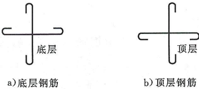
图 4.3.5-1 平面图中的双层钢筋
