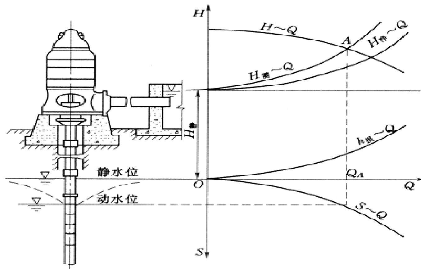
图 3-4 井泵工作点的确定
