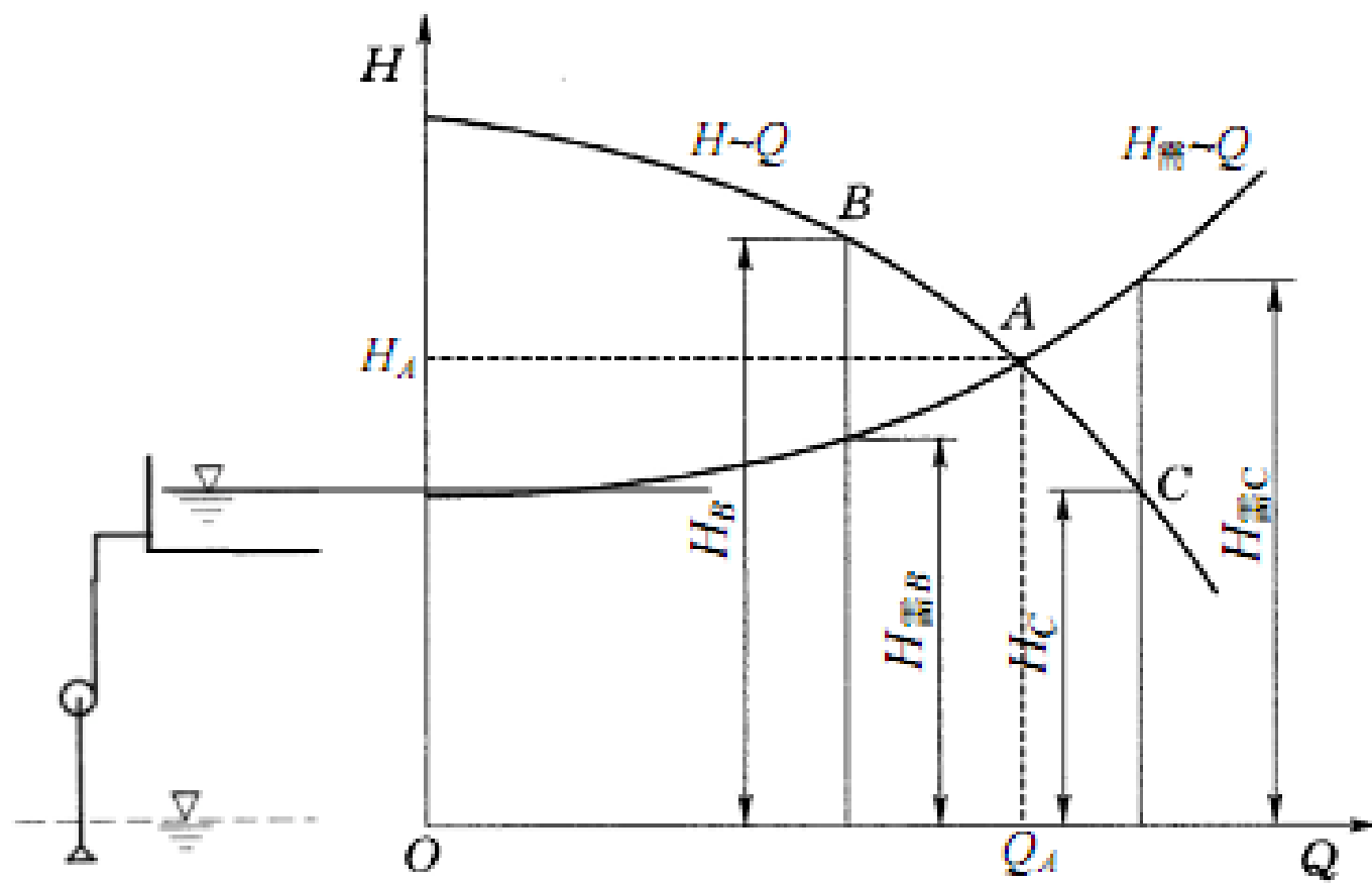
图 3-2 图解法确定水泵工作点
