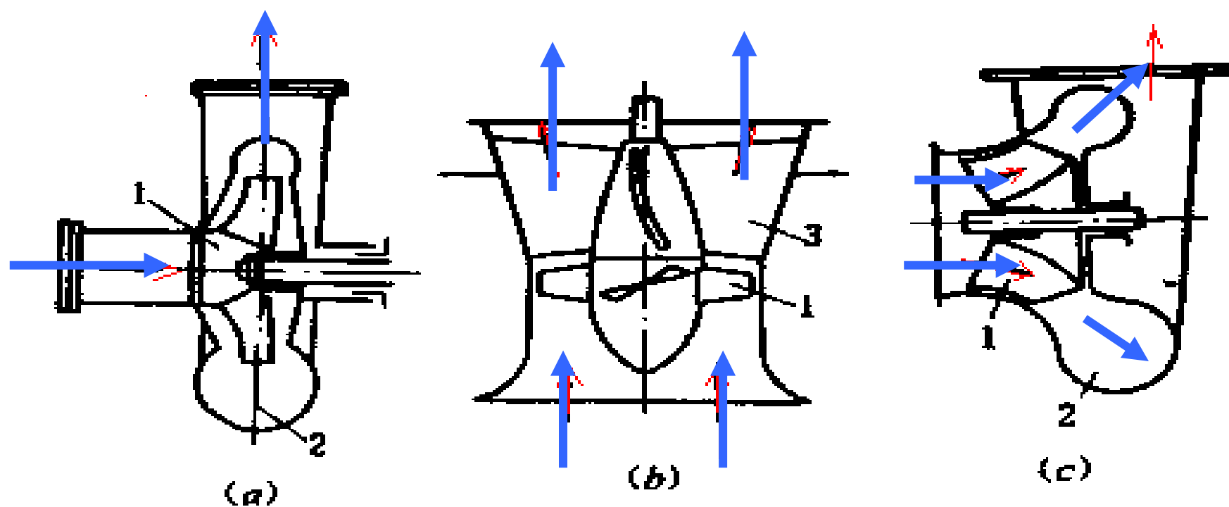
图 1-1 叶片式泵
