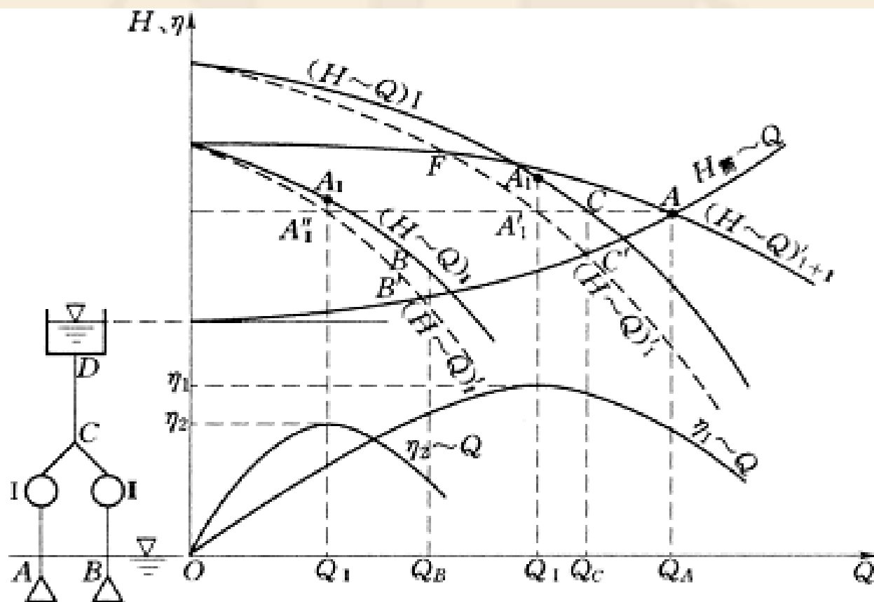
图 3-7 不同型号水泵并联运行工作点的确定
